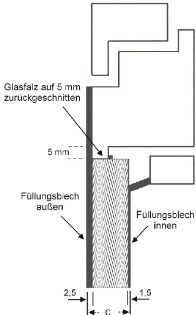
Schnitt Detailansicht ( Vertikal )
